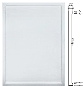
45°Beveled Door
